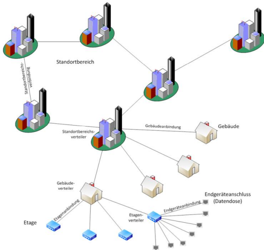
Abbildung 2 – Netzstruktur (schematisch)
