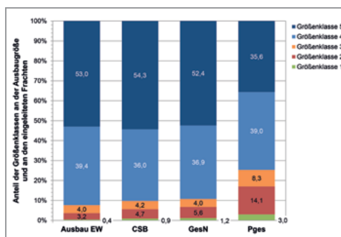
Abbildung 2: Prozentuale Anteile der Ausbau-EW und der eingeleiteten Frachten nach Kläranlagen-Größenklassen
