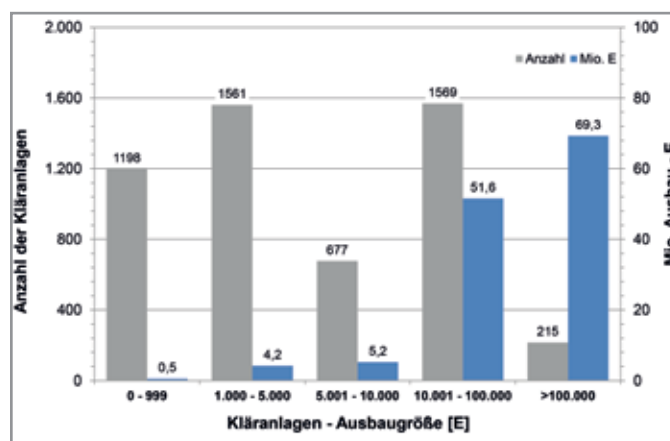
Abbildung 1: Anzahl und Ausbaupgrößen der am DWA-Leistungsnachweis 2020 beteiligten Kläranlagen nach Größenklassen
