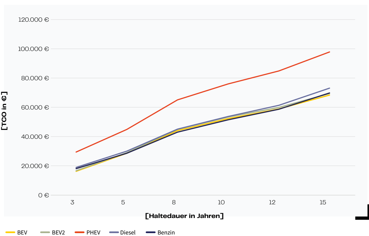
Abbildung 4: TCO-Vergleich von Antriebsoptionen in der Pkw Kleinwagenklasse in Abhängigkeit der Haltedauer
