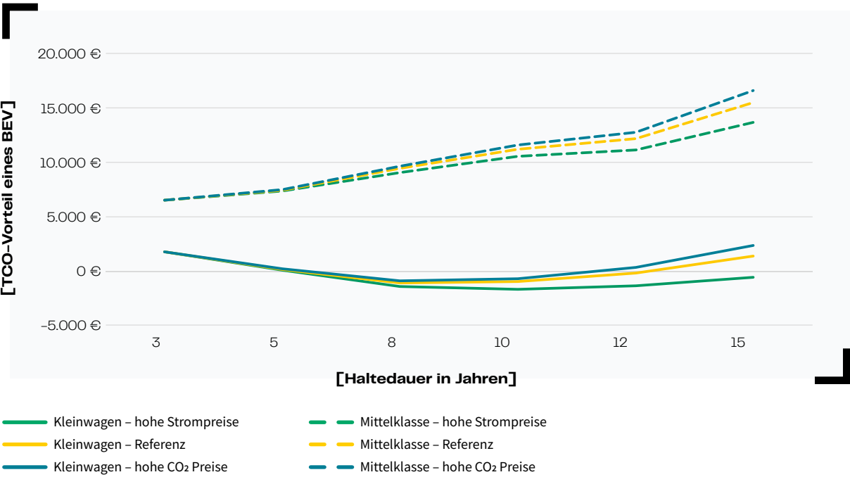
Abbildung 9: TCO-Vergleich des Kostenvorteils von BEV gegenüber Benzinern in Abhängigkeit der Entwicklung der Strom- und Benzinpreise
