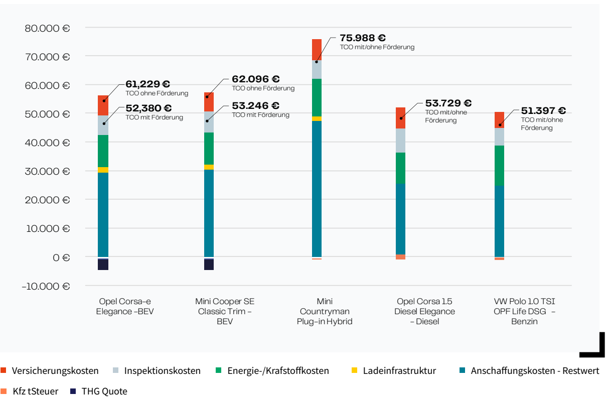
Abbildung 7: Anteile der TCO bei den Antriebsoptionen am Beispiel der Pkw Kleinwagenklasse
